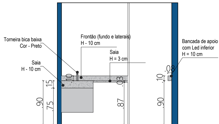
Vista 01 - Banho social Sem escala
