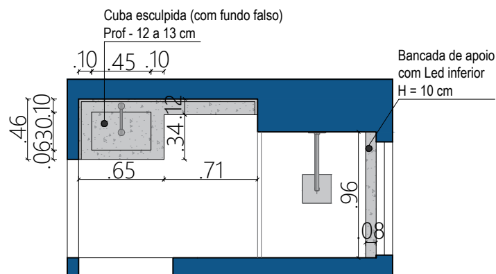
Planta baixa - Banho social Sem escala
